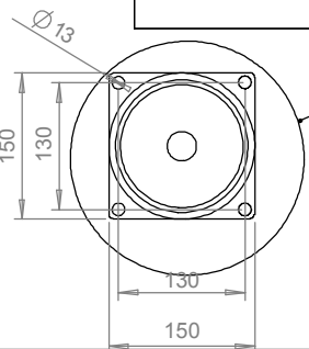
Détail des systèmes d'acrochage de sangle
