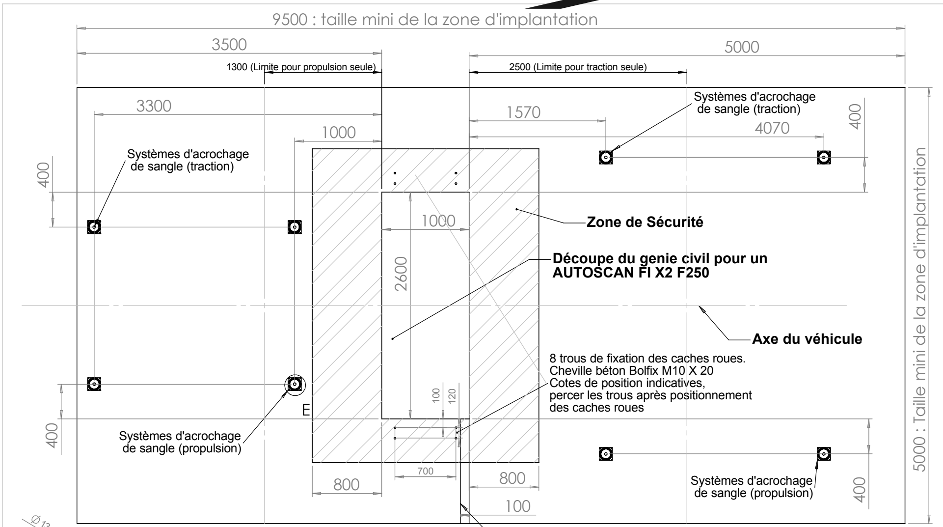
Détail des systèmes d'acrochage de sangle
